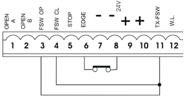
Connexion d'un dispositif de sécurité "bord"
