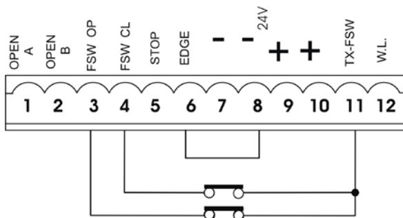
Connexion d'un dispositif de sécurité en fermeture et d'un dispositif de sécurité en ouverture
